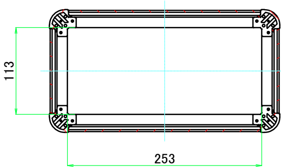
C-C ( 1 : 5 )
