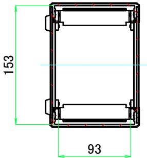
A-A ( 1 : 5 )
